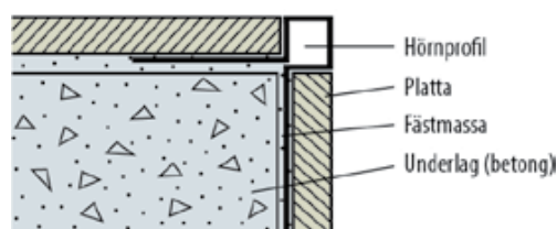
Horizontalsnitt
