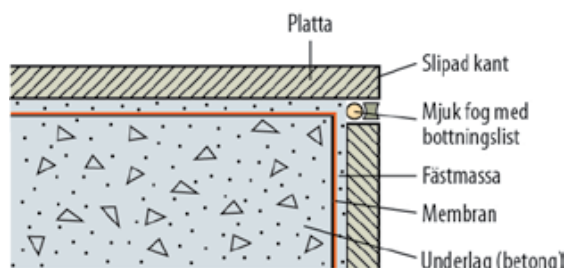
Horizontalsnitt
