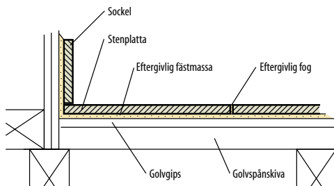
Alt B: Montering i fästmassa på träkonstruktion
